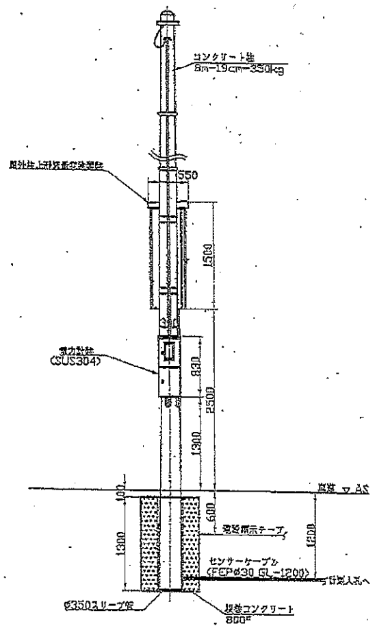
側面図
