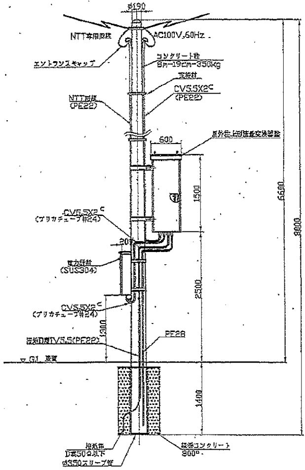
正面図
