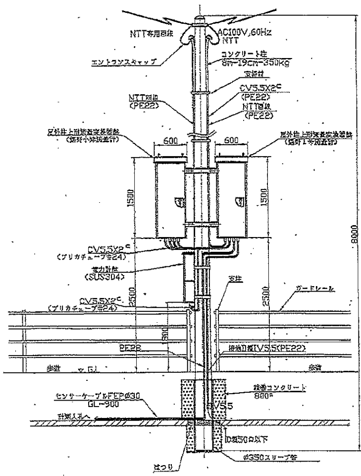
正面図
