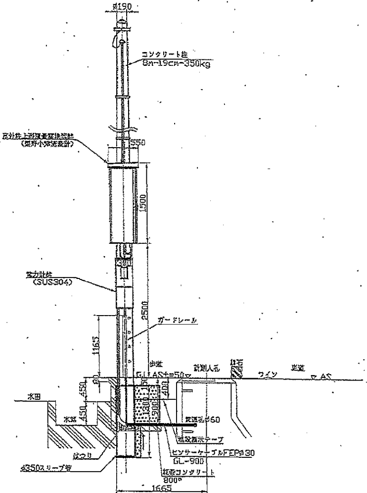
側面図
