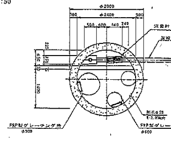
断面C-C
