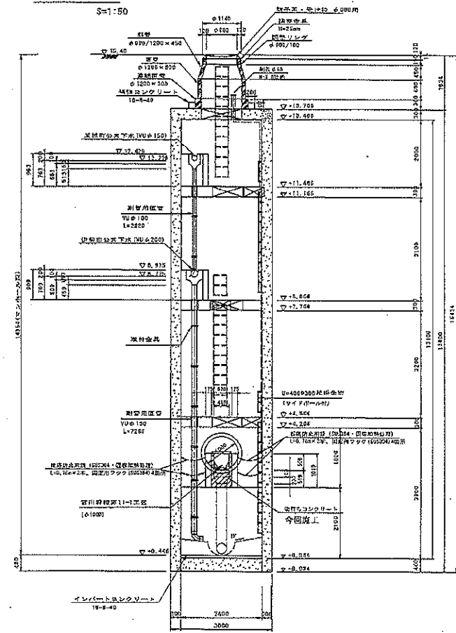
断面B-B
