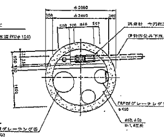
断面E-E
