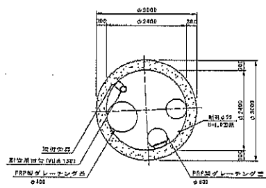
断面E-E
