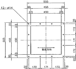
⑩ 出入口フランジ (S=1/10)
