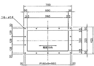
⑨ 突入口フランジ (S=1/10)
