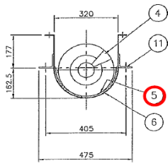
⑤ U-320 ロール (S=1/10)
