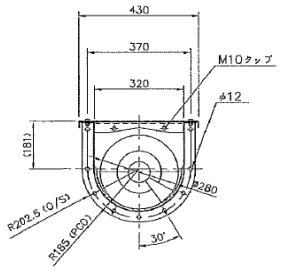
⑧ U-320 フランジ (S=1/10)
