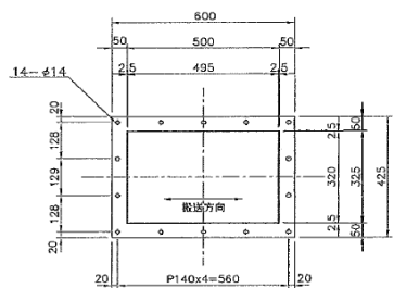
inlet flange (S=1/10) 9
