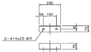
⑪ ロボートブacket (S=1/10)
