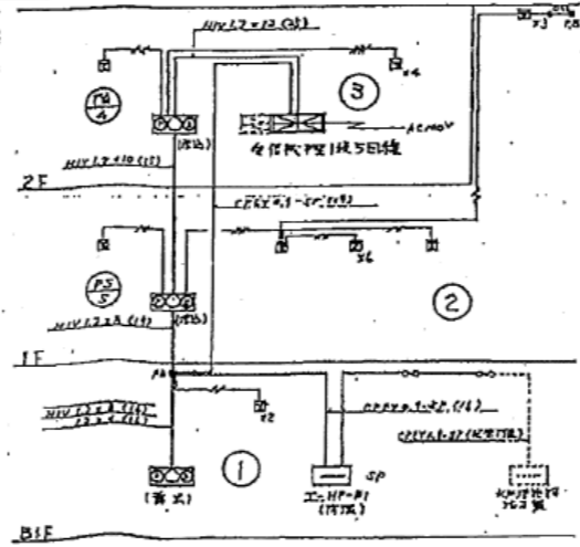
自動火災探知設備系統図
