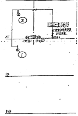
防煙探知設備系統図
