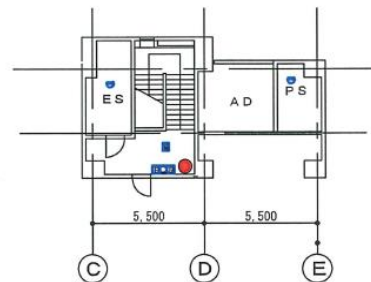
塔屋平面図1:200
