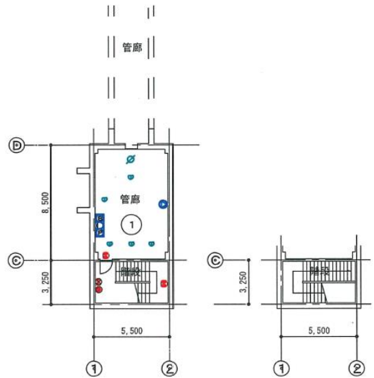
管理本館地下1階平面図 1:200
