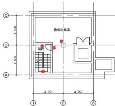
B 1階平面図1:200
