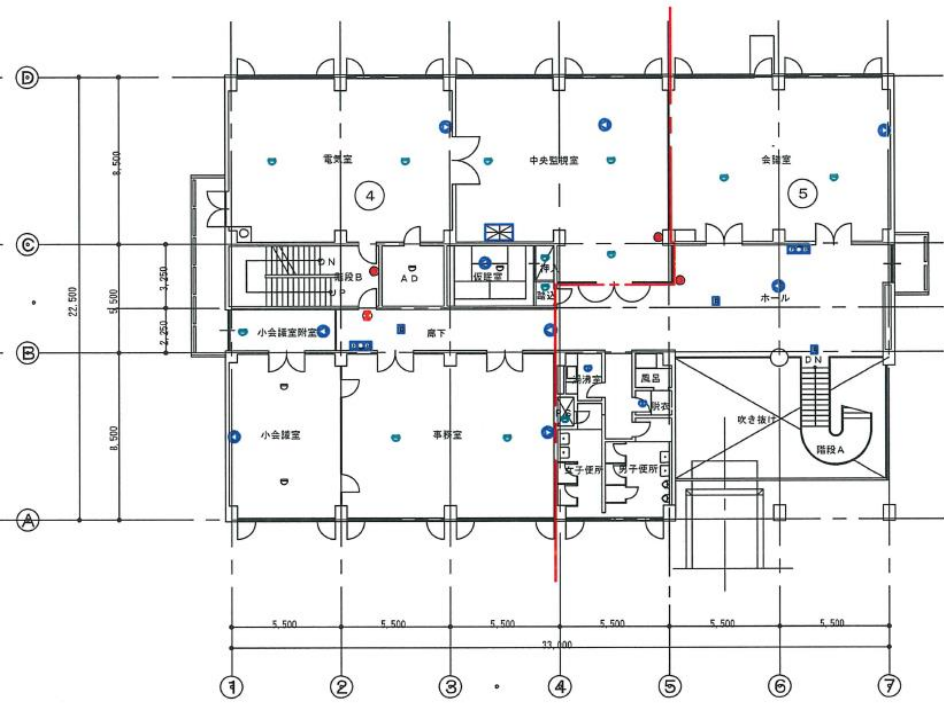
管理本館 2階平面図 1:200
