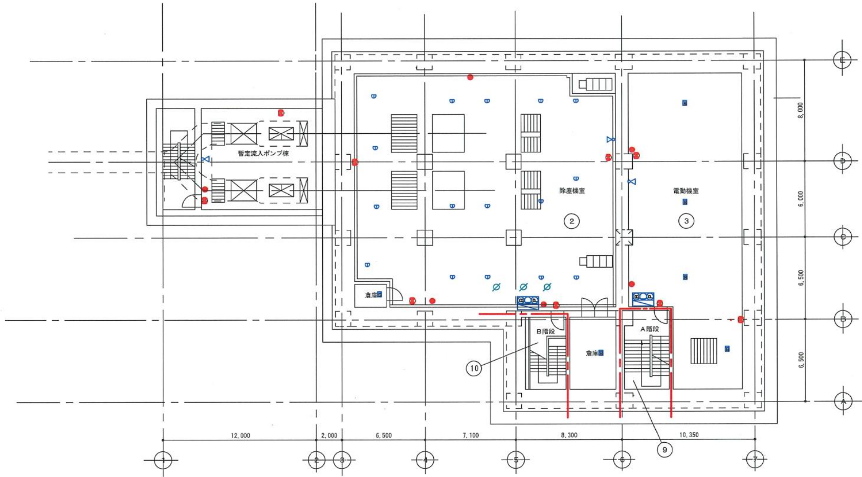
B 2 階平面図 S = 1:200
