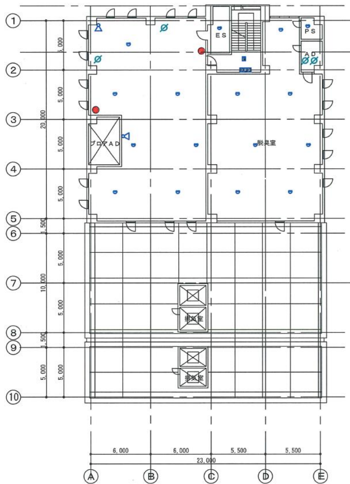
3階平面図1:200
