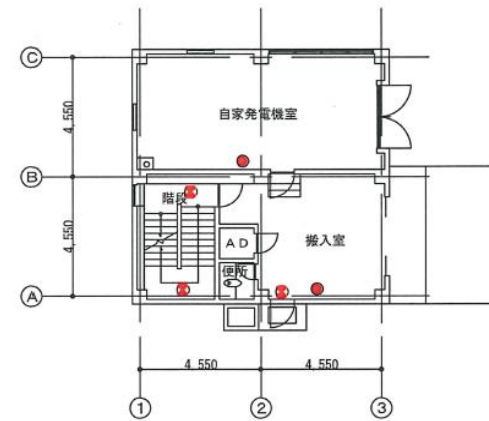
1階平面図1:200
