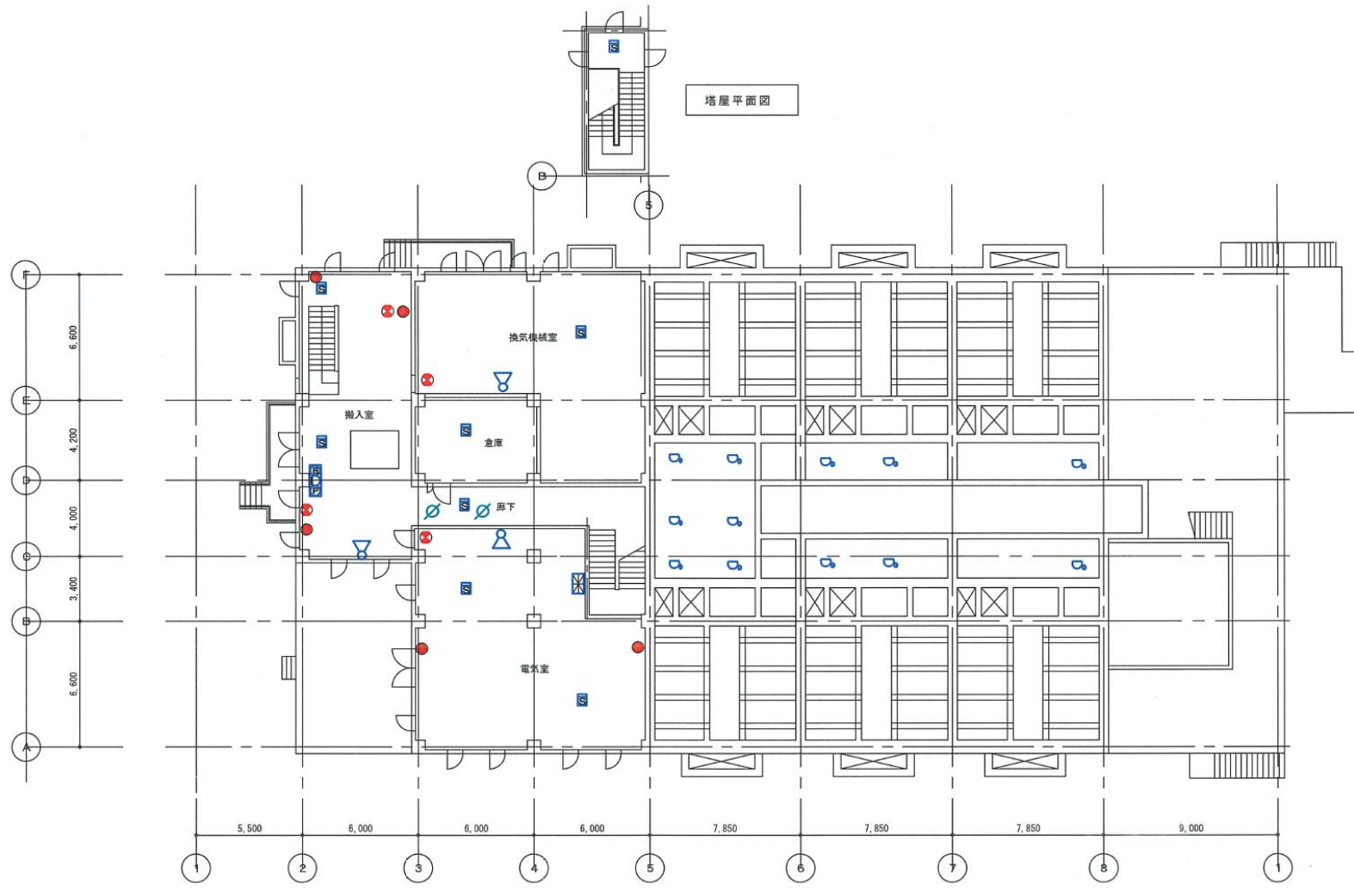
1階 平面図 1:200
