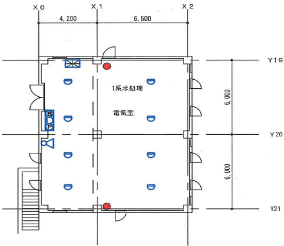
1系水処理電気室（1系水処理上部）1:200
