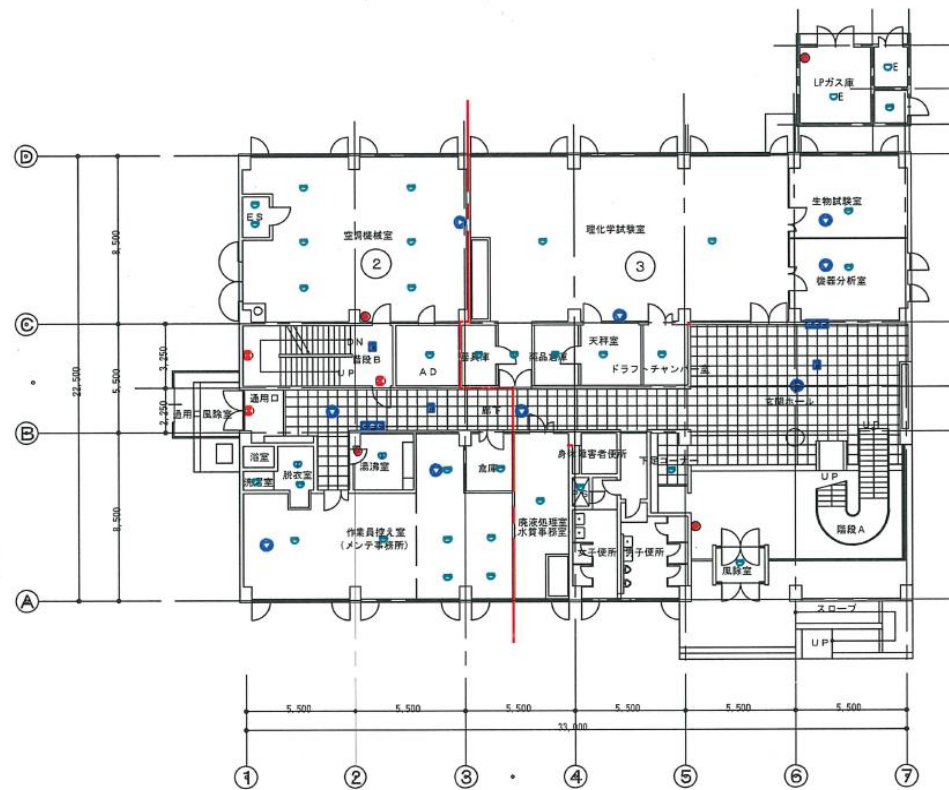
管理本館1階平面図 1:200
