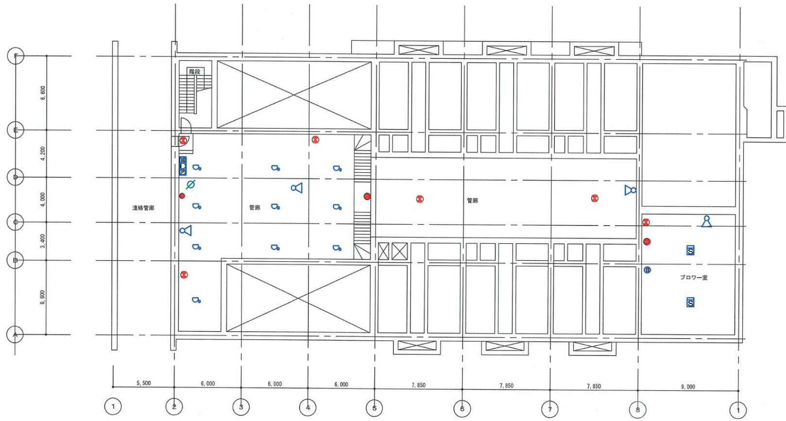
B1階 平面図 1:200
