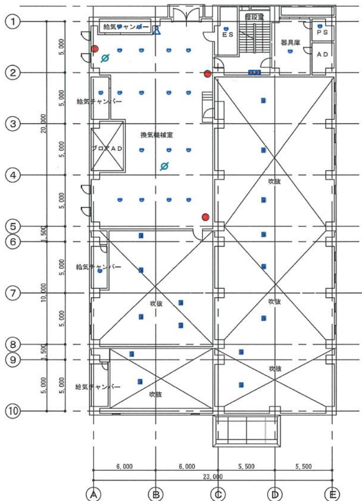
2階平面図1:200
