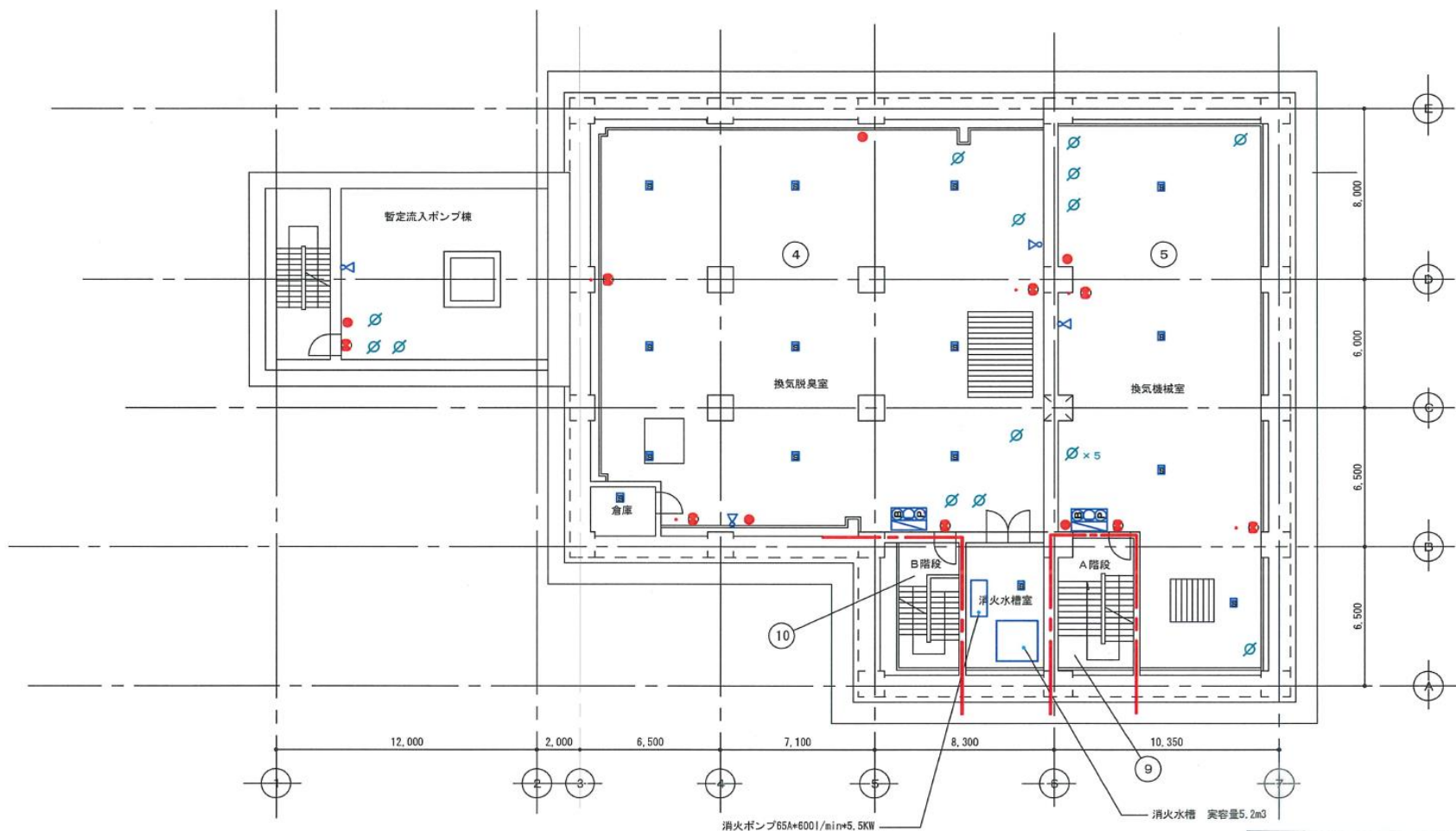
B 1 階平面図 S = 1:200
