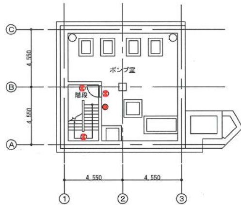
B 2階平面図1:200
