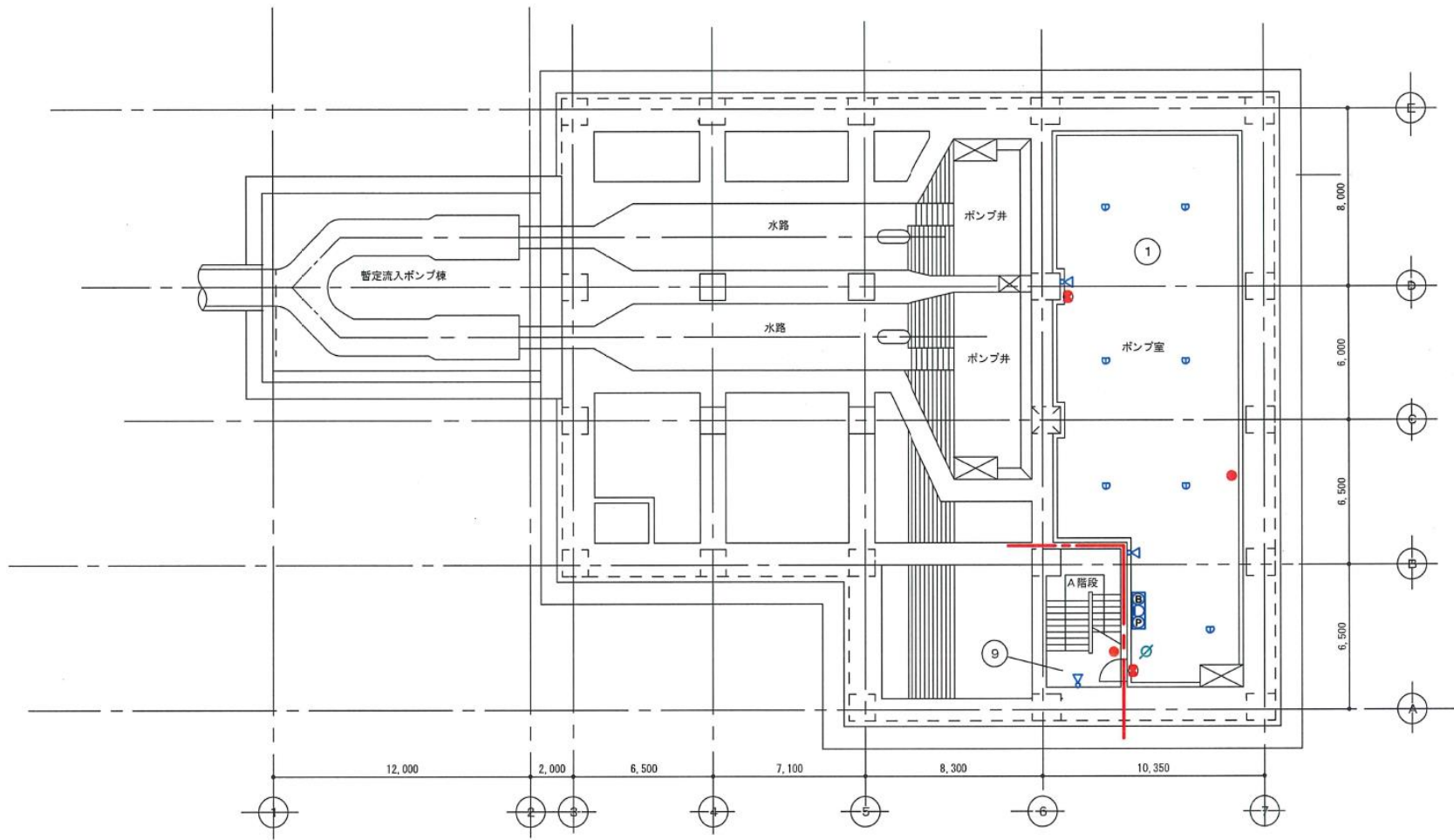
B 3 階平面図 S = 1:200
