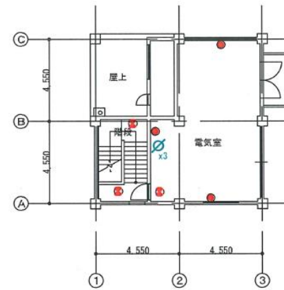
2階平面図1:200
