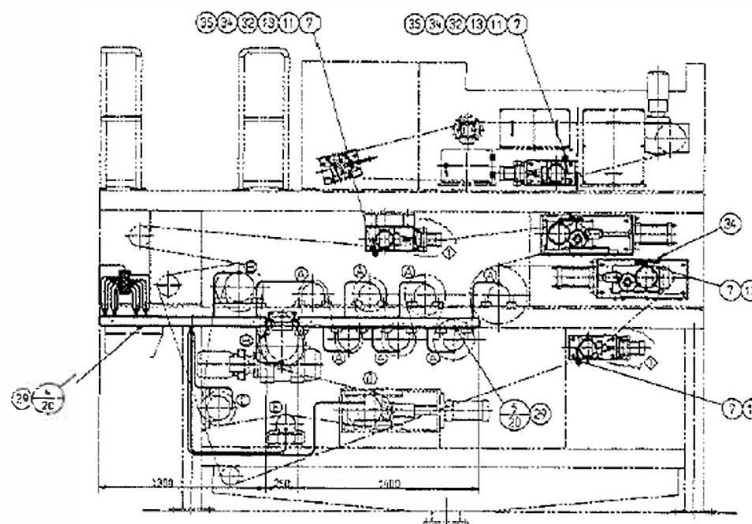
図 2-1-10 (S=1/2)
