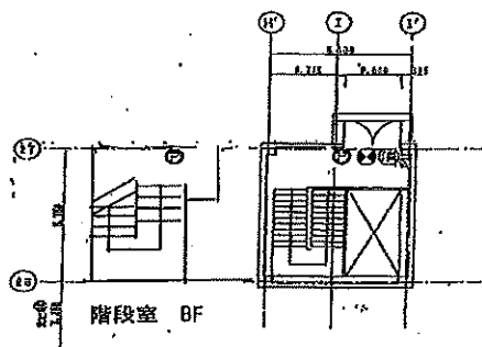
階段室 BF 図面番号: 1月字002 P-11(12)
