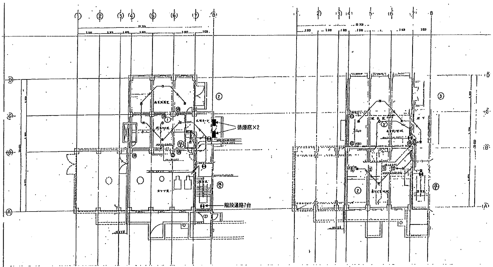
1階平面図 1/100
