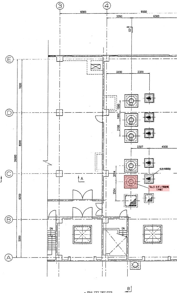
1階平面図
