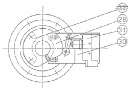
A-A' 矢視図
