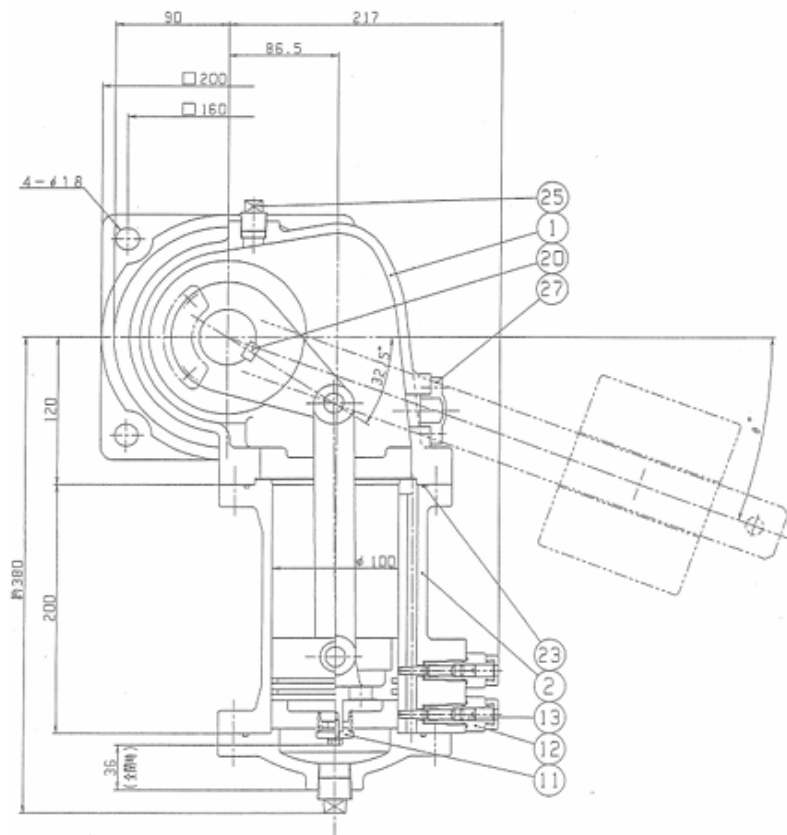
A-A' 矢視図
